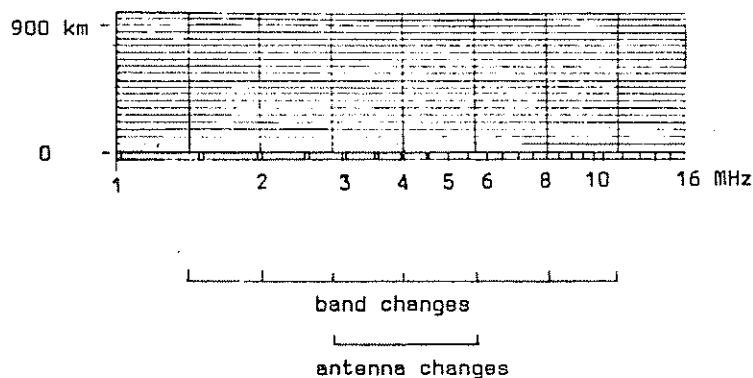
Ionogram parameters
