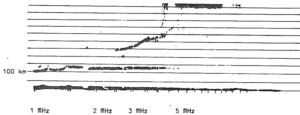
Fig. 1. Simultaneous ionograms 20.6.1973. 20.40 LT, Sodankylä
